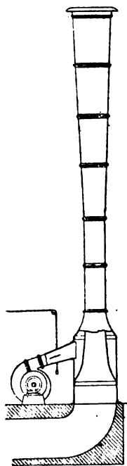
Fig. 69. — Tirage par entraînement système Prat.
